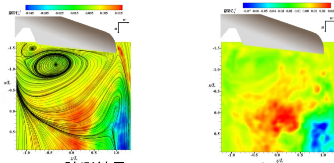
(a) PIV計測結果
